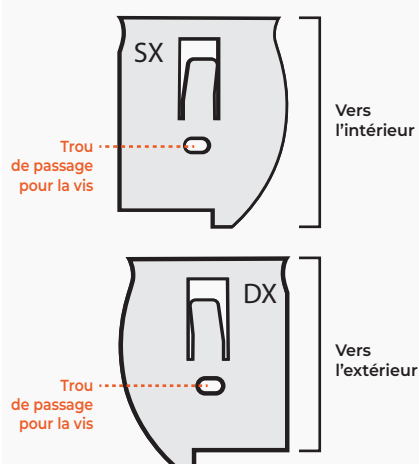
Schéma des supports de bloc
