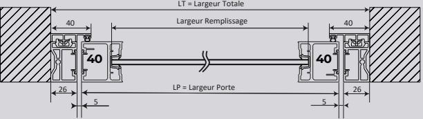
Porte 40/66
