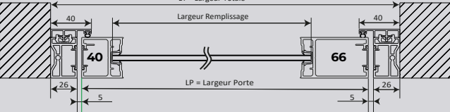
Porte 40/66
