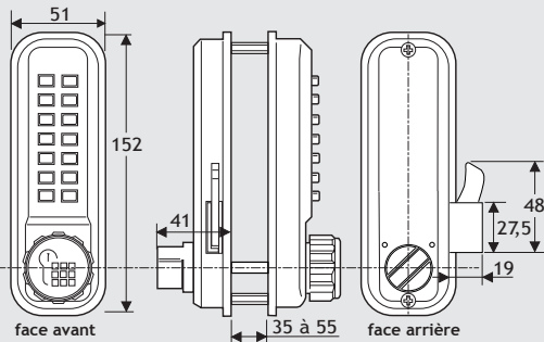
MODÈLE U2500 pêne en applique à crochet
