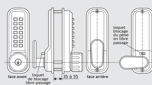
MODÈLE U2435 CS pêne demi-tour à larder, libre passage et clé de secours
