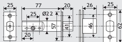
• pêne dormant à larder
