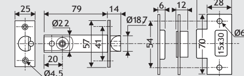
• pêne demi-tour à larder
