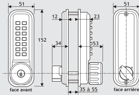
MODÈLE U2210 CS pêne dormant à larder et clé de secours MODÈLE U2230 CS pêne demi-tour à larder et clé de secours
