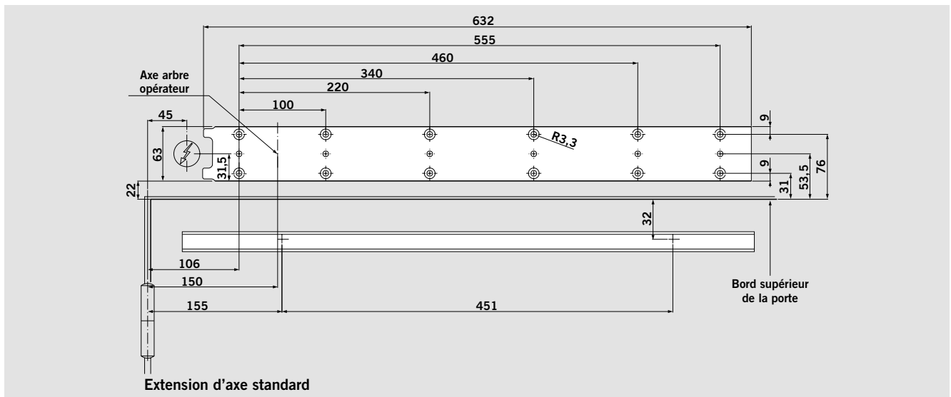
Gabarit de perçage : Capot standard, montage tirant, axe du coulisseau de glissière 25 mm
