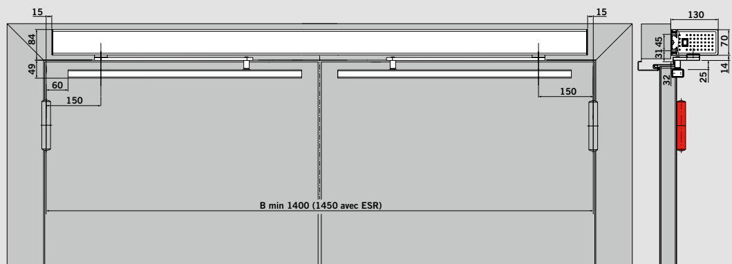
Extention d'axe standard
