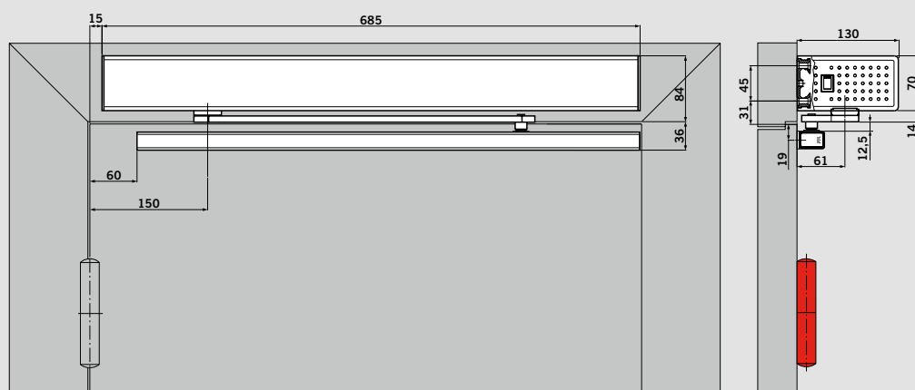
Extention d'axe standard
