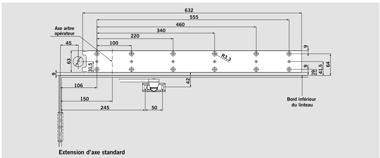
Gabarit de perçage : Capot standard, montage poussant
