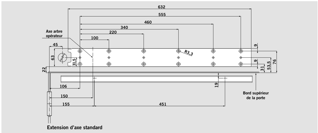
Gabarit de perçage : Capot standard, montage tirant, axe du coulisseau de glissière 12,5 mm
