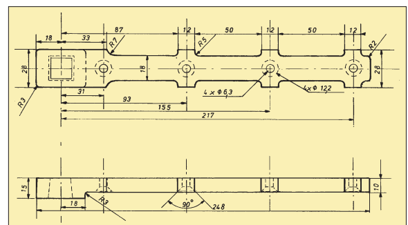
Bras inférieur B carré, bronze aluminium.
