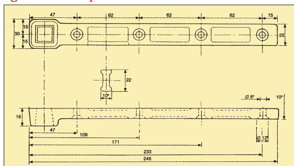
Bras inférieur A bis carré, bronze aluminium.
