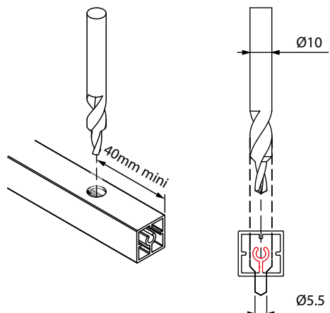
Foret étagé Ø10-5.5
