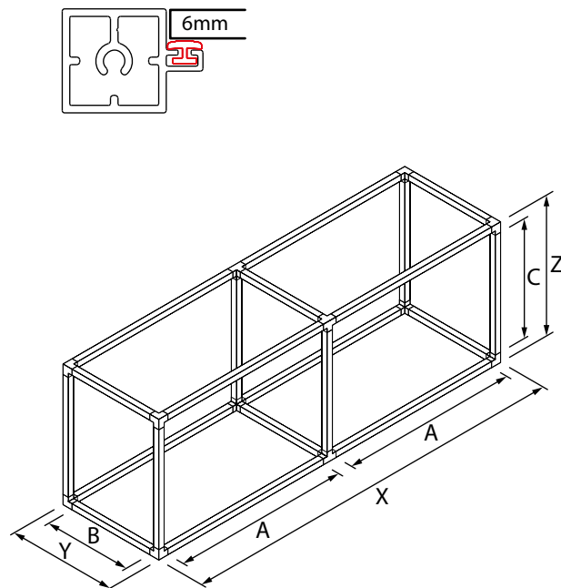
Profil carré épaisseur 6-8mm + joint plat
