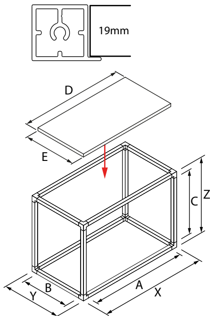
Profil carré épaisseur 19mm
