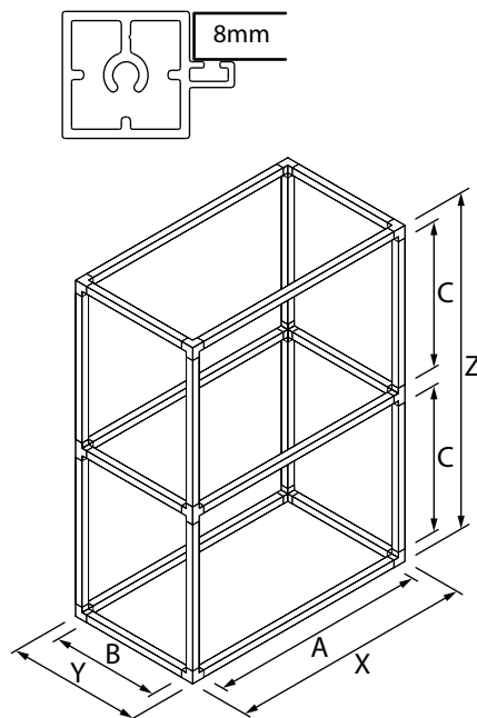
Profil carré épaisseur 6-8mm
