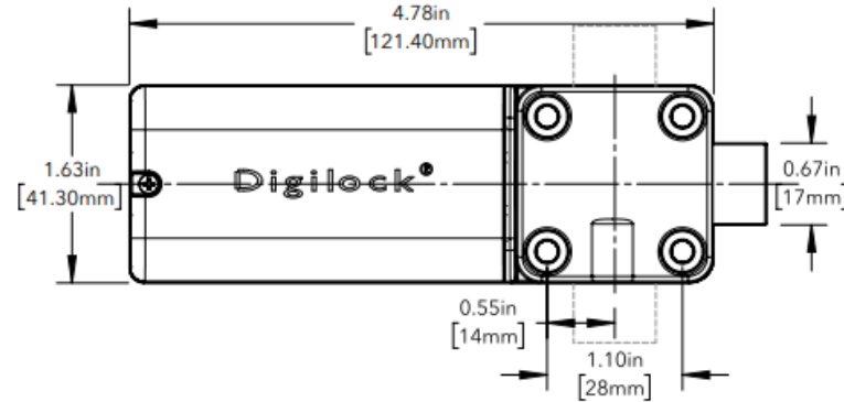
VUE LATÉRALE
