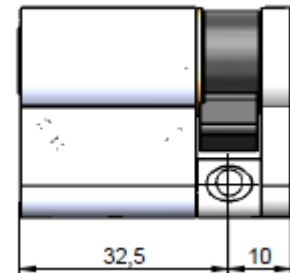
Cylindre simple
