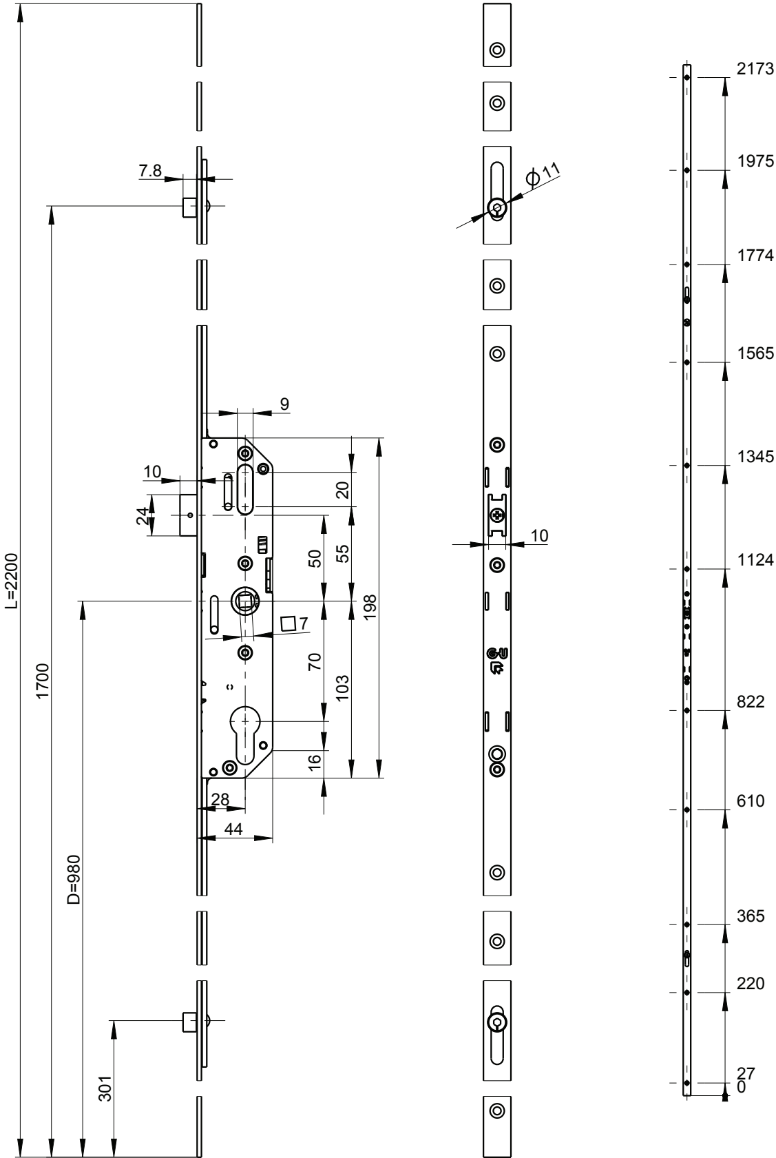
Crémone gauche représentée en position ouverture
