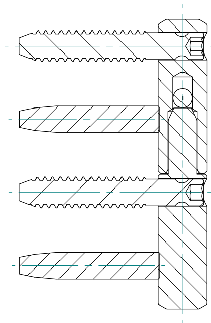
SEZIONE B-B
