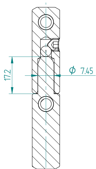
SEZIONE A-A
