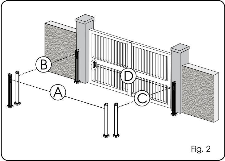
La fig. 2 illustre un automate pour portail battant à 2 vantaux avec les faisceaux de couverture des photocellules:
