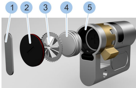
Fig. 82: Insérer les piles
