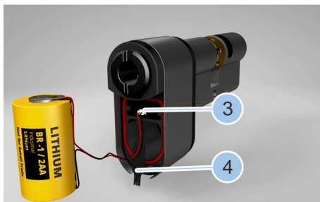
Fig. 92: Retirer la pile
