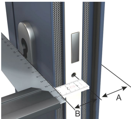
Fig. 26: Mesurer le cylindre
