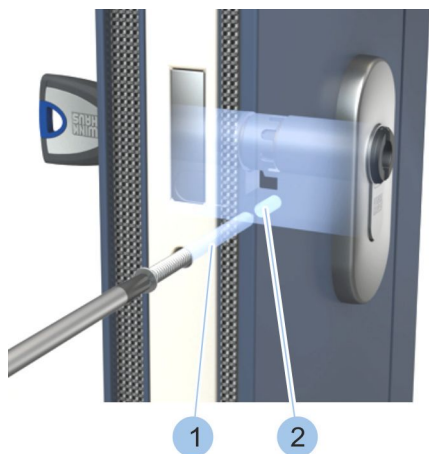
Fig. 34: Visser la vis de fixation
