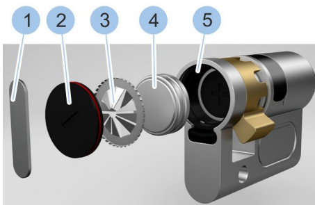
Fig. 81: Retirer les piles
