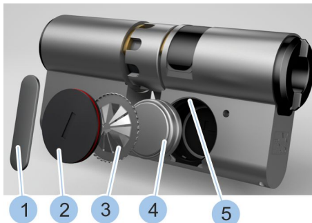
Fig. 79: Insérer les piles
