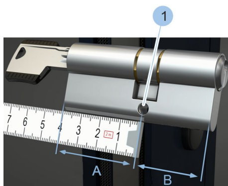
Fig. 24: Mesurer l'ancien cylindre
