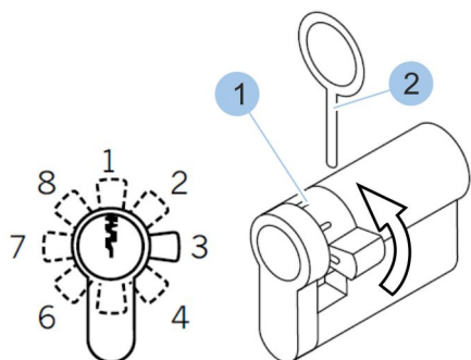
Fig. 31: Modifier la position du panneton
