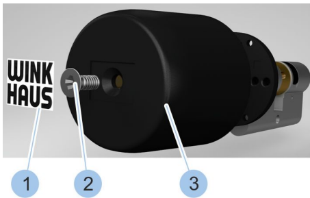
Fig. 84: Retirer le bouton
