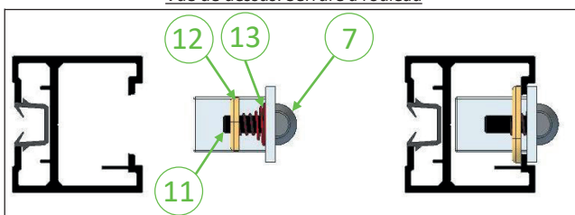
Vue de dessus: Serrure à rouleau
