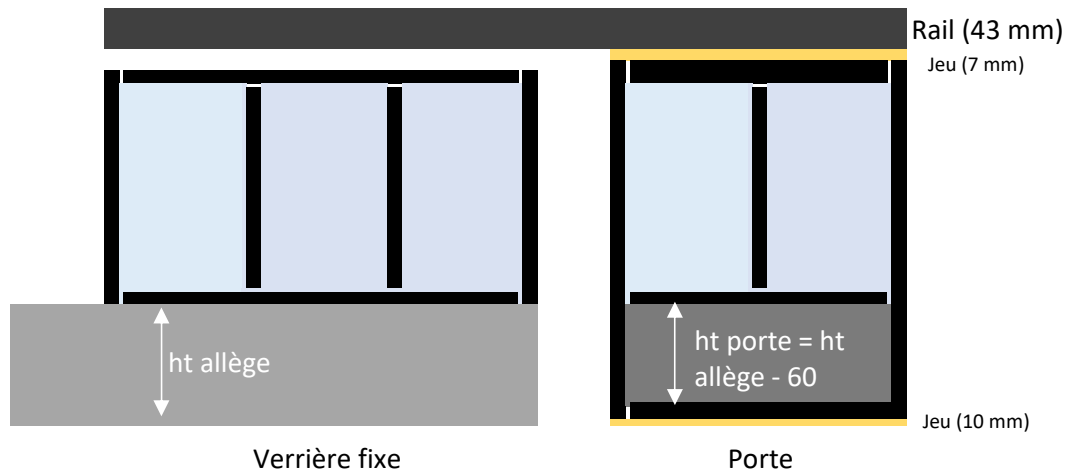
Cas 2 : verrière sur allège
