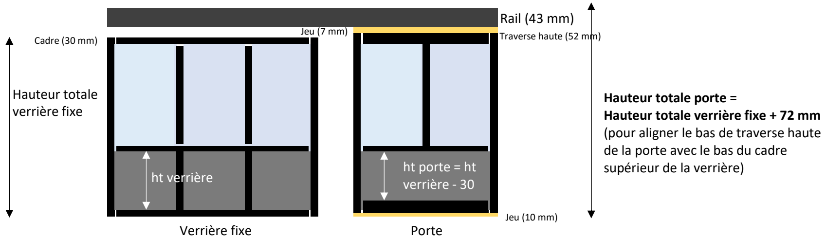
Cas 1 : verrière avec soubassement
