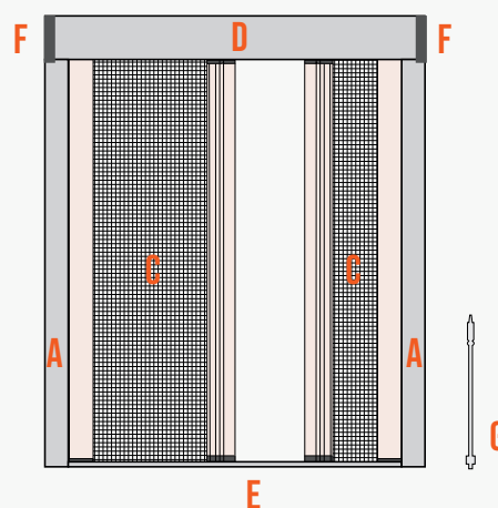
Moustiquaire latérale 2 vantaux
